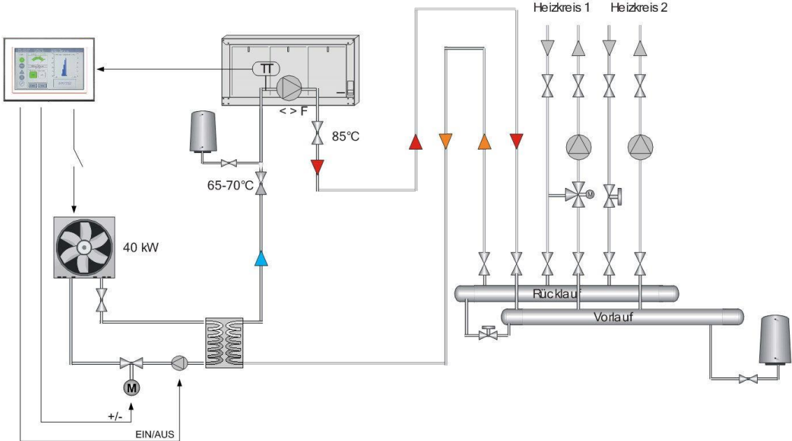
Abbildung 8: Anschlussbeispiel mit Notkühlung
