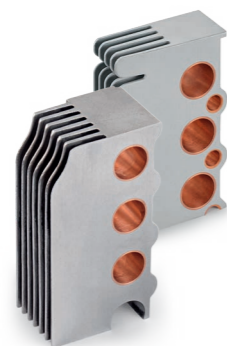
TopGas®-Wärmetauscher: Cleverer Materialmix aus leitfähigem Aluminium und korrosionsbeständigem Kupfer. Der TopGas® combi (hinten) hat einen zusätzlichen Kupfer-Wasserkanal für die Warmwasserbereitung.
