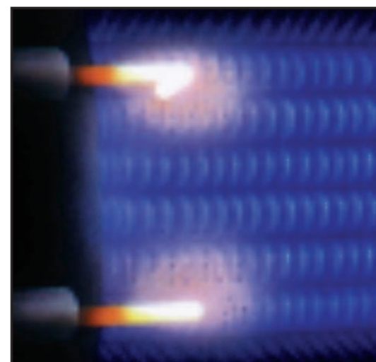
Im Flächenbrenner wird das Gas-Luft-Gemisch auf der Oberfläche eines Metallgewebes entzündet und verbrennt leise und nahezu flammenlos. Die Wärme wird größtenteils als Infrarotstrahlung abgegeben. Die gleichmäßige Verbrennungstemperatur liegt dabei in einem optimalen Bereich und ermöglicht minimale Schadstoff-Emissionen.
